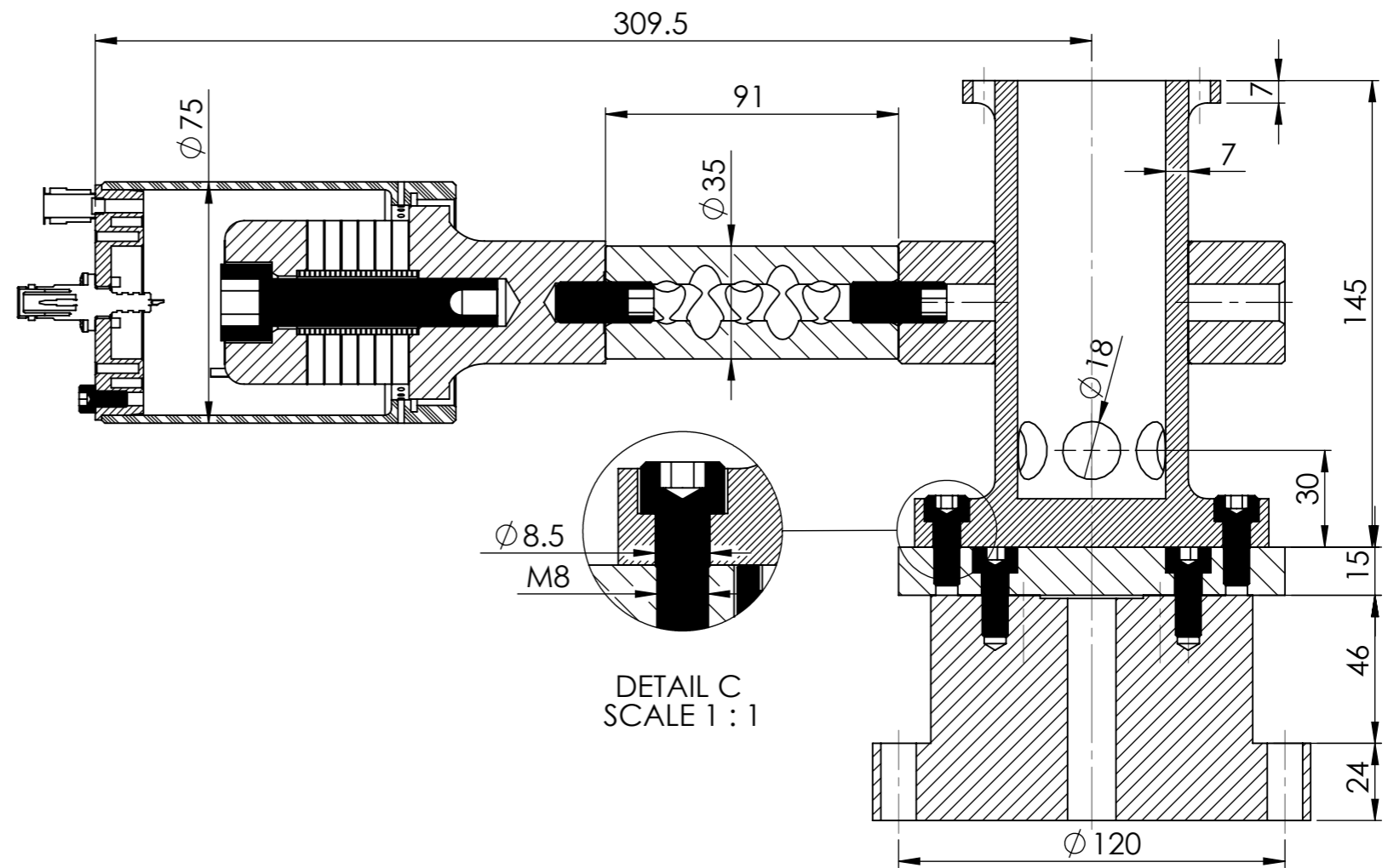
SECTION A-A
